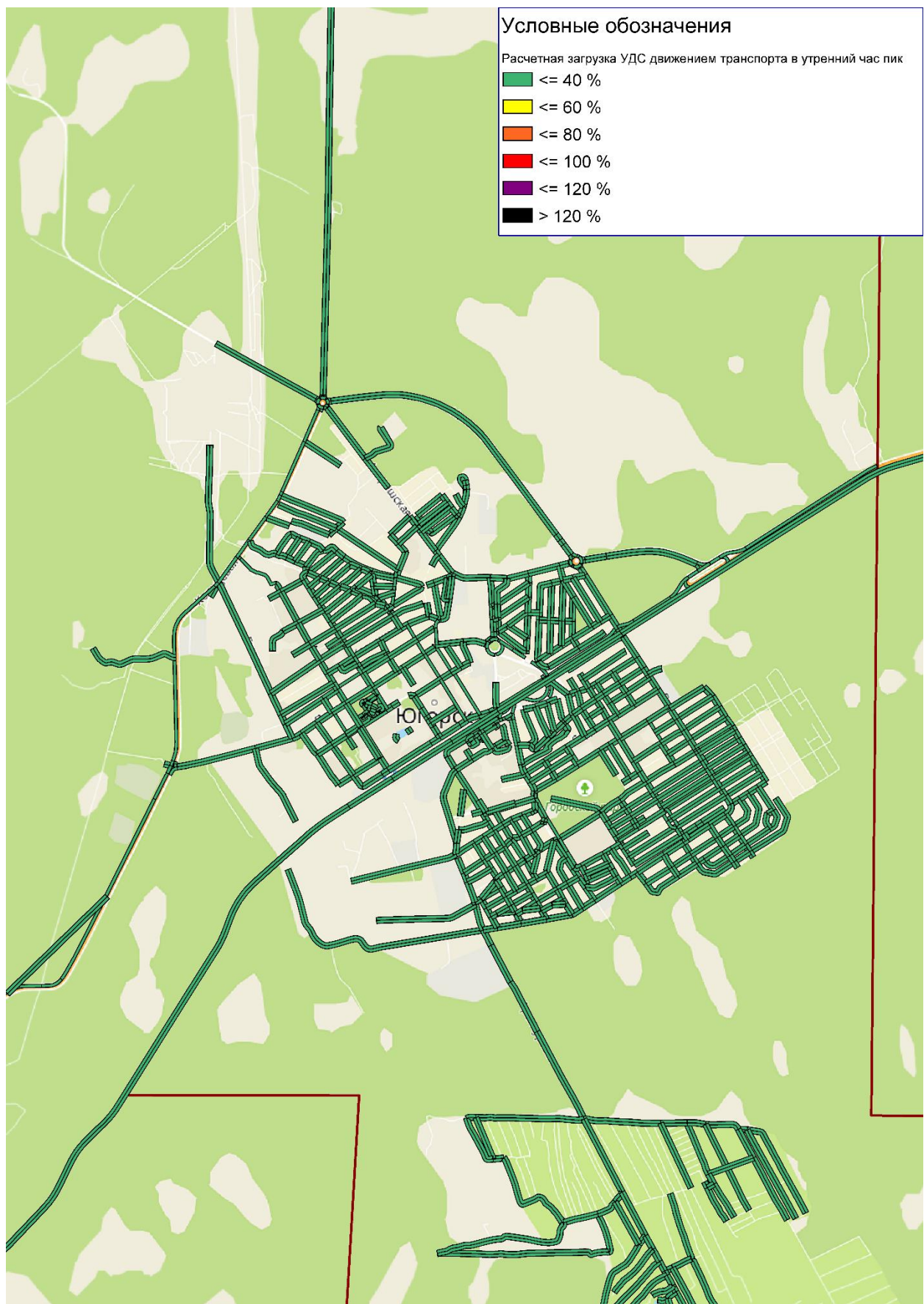
Рисунок 8 – Картограмма расчетной загрузки УДС движением транспортных потоков в час пик
